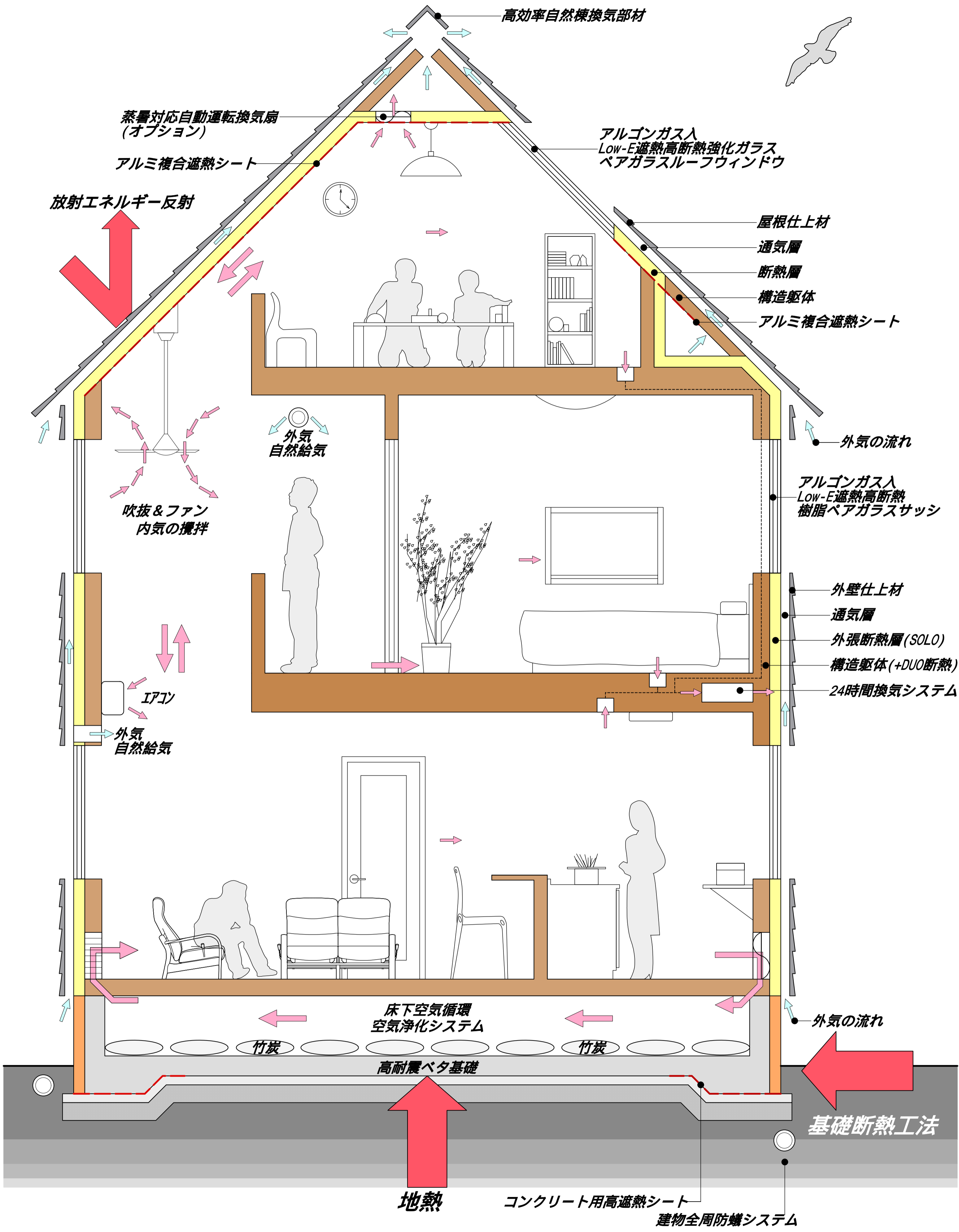
EHCシステム概念図 Earth Comfort & Human Comfort System
